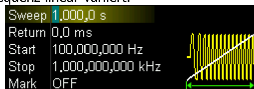
Bild 2-7 Linearer Sweep
