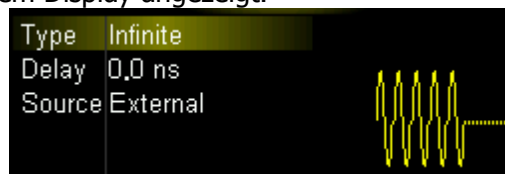
Bild 2-11 Unendlicher Burst
