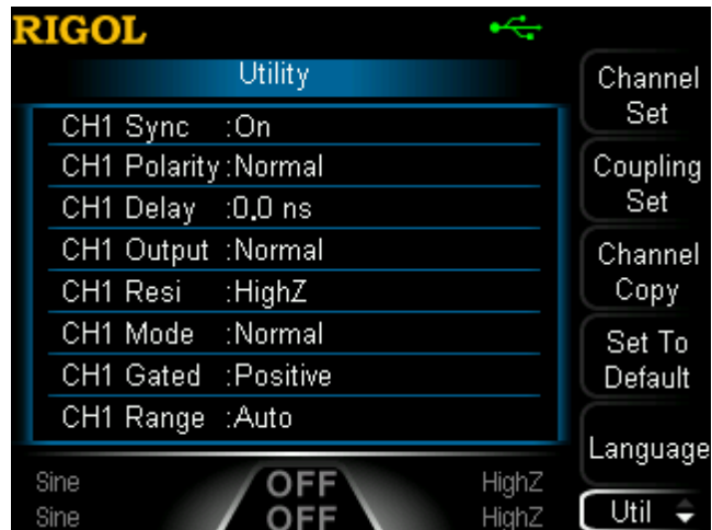
Bild 2-19 Utility Schnittstelle
