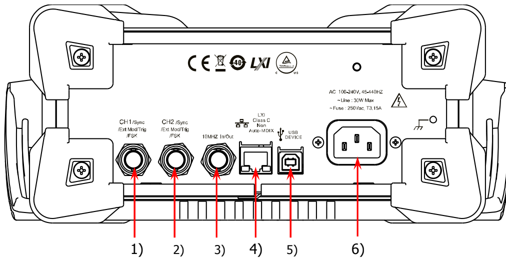
Bild 1-2 Rückseite
