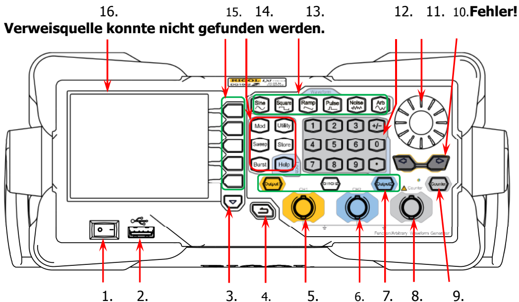
Bild 1-1 Front Panel
