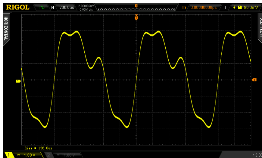
Bild 2-6 Harmonische Schwingung
